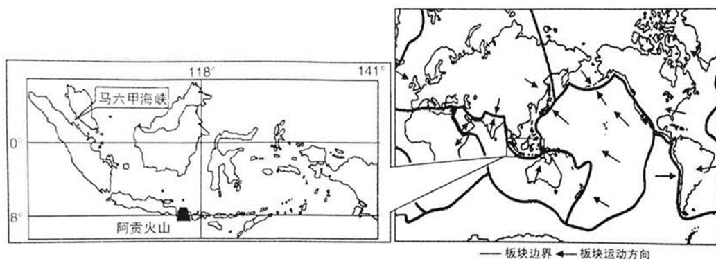
图2 阿贡火山位置示意图
